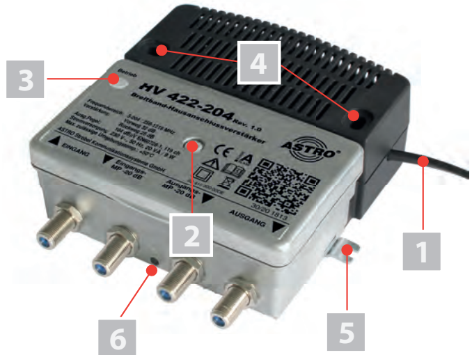
Bild 1: Verstärker HV 422-204
