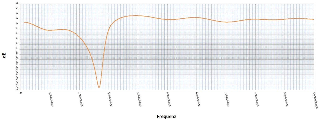
EOC2000 Einfügedämpfung
